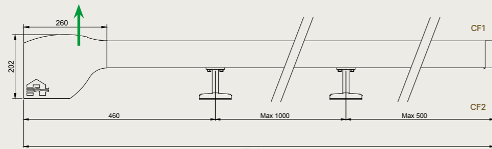
Vue latérale
