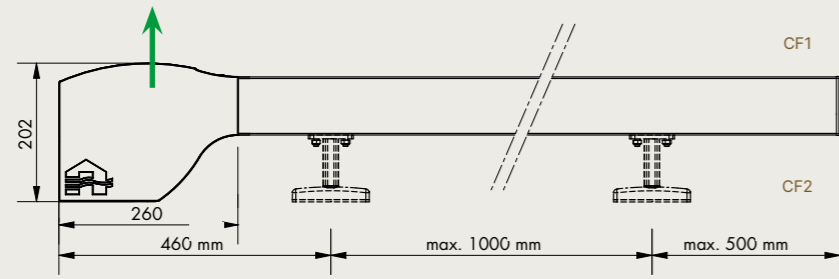
Vue latérale
