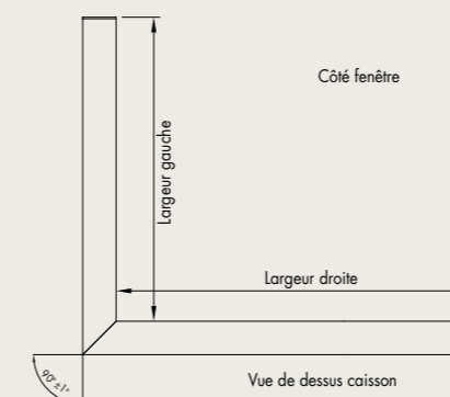
VUE DE DESSUS DU CAISSON
