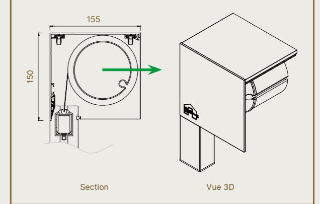
Fixscreen® 150 - Caisson
