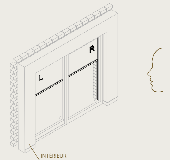
Fixscreen® M 4/M 7B Fixscreen® / Fixvent® Mono AK/UT
