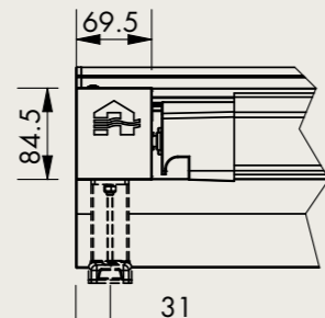
Vue avant
