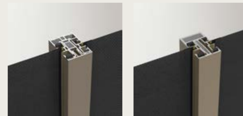
C.40 — Coulisse d'accouplement pour M 7A
