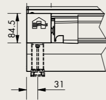
Vue avant
