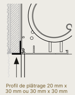
Profil de plâtrage
