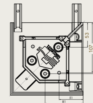
Équerre d'angle (position des trous de forage)
